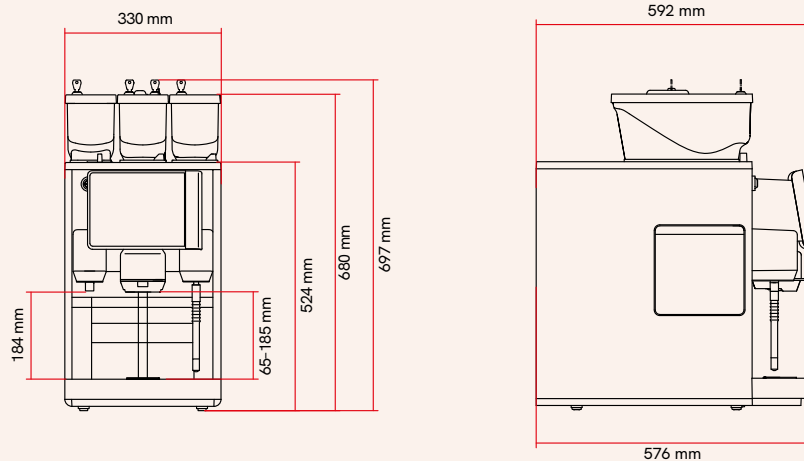
Schaerer Coffee Skye Frontansicht/ Seitenansicht rechts
